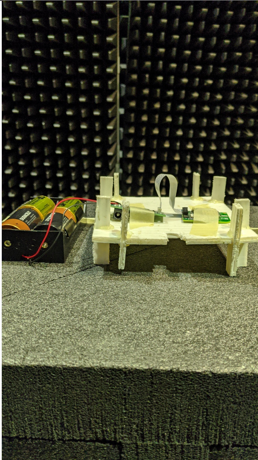
EUT Flat
