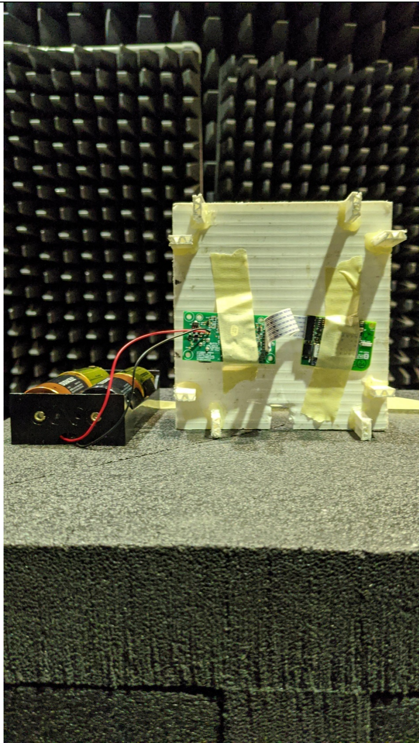
EUT Vertical
