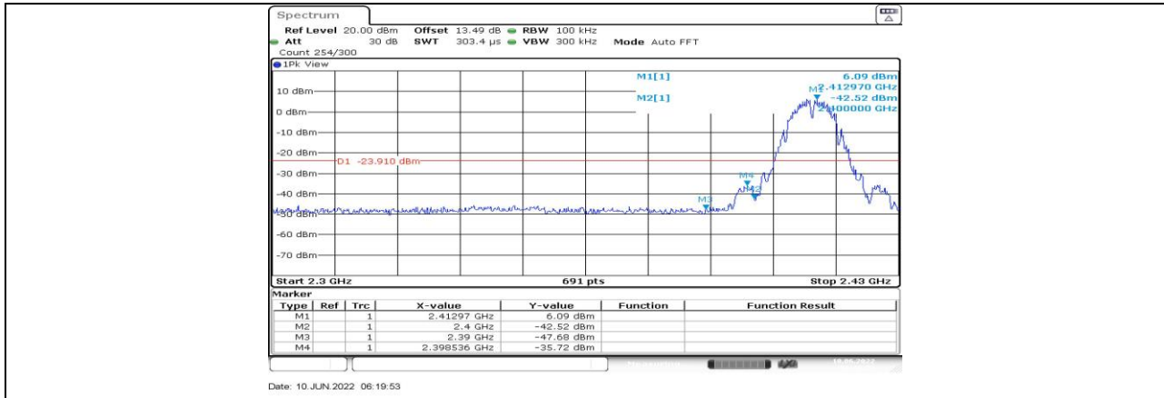
11B_Ant1_Low_2412
