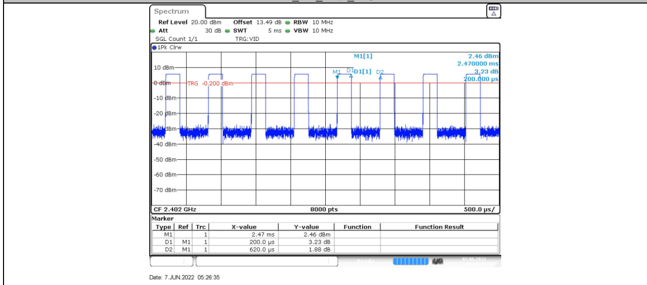
BLE_2M_Ant1_2402
