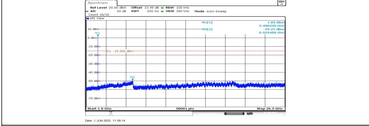
BLE_2M_Ant1_2480_1000~26500
