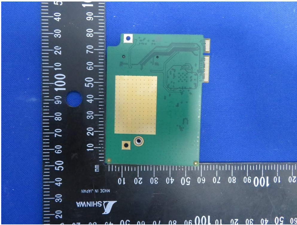
(13) EUT Photo
