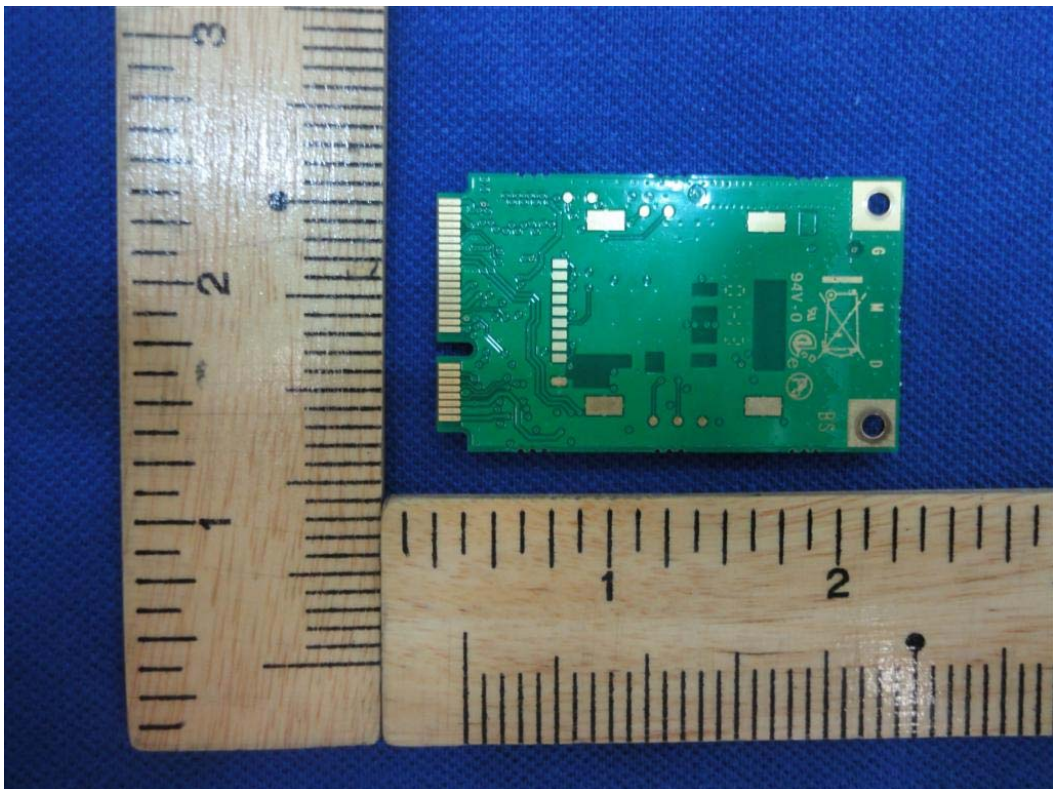
10) EUT Photo
