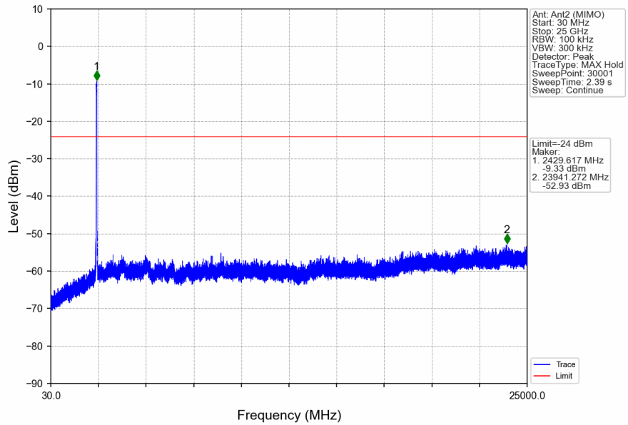
802.11n(HT40)_LCH_2422MHz_Ant2 (MIMO)_NTNV
