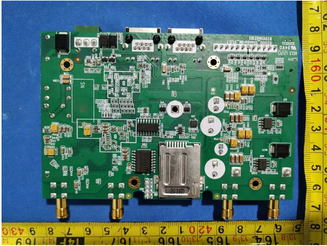
WWAN Module
