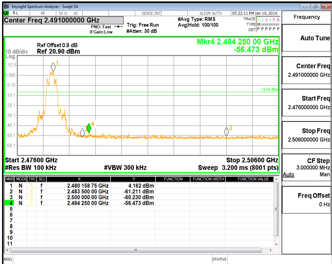
(Plot 4.9.2 D2: Right Band edge hopping off @ 8DPSK)
