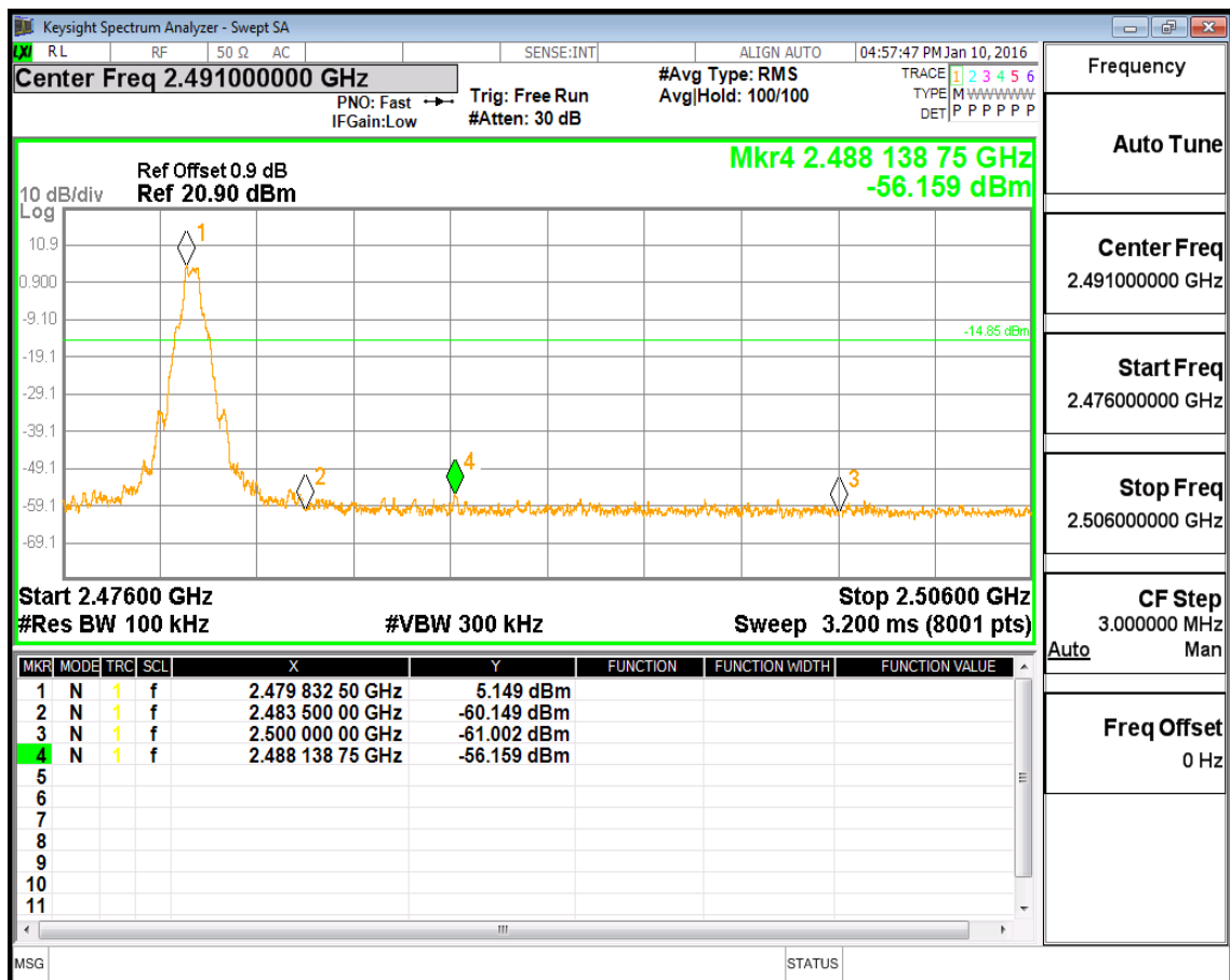
(Plot 4.9.1 D2: Right Band edge hopping off @ GFSK)
