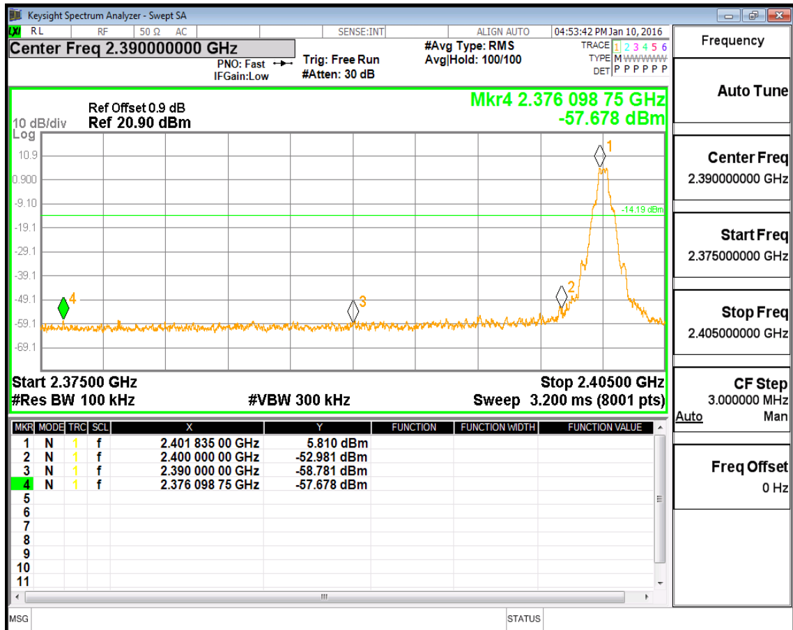
(Plot 4.9.1 D1: Left Band edge hopping off @ GFSK)
