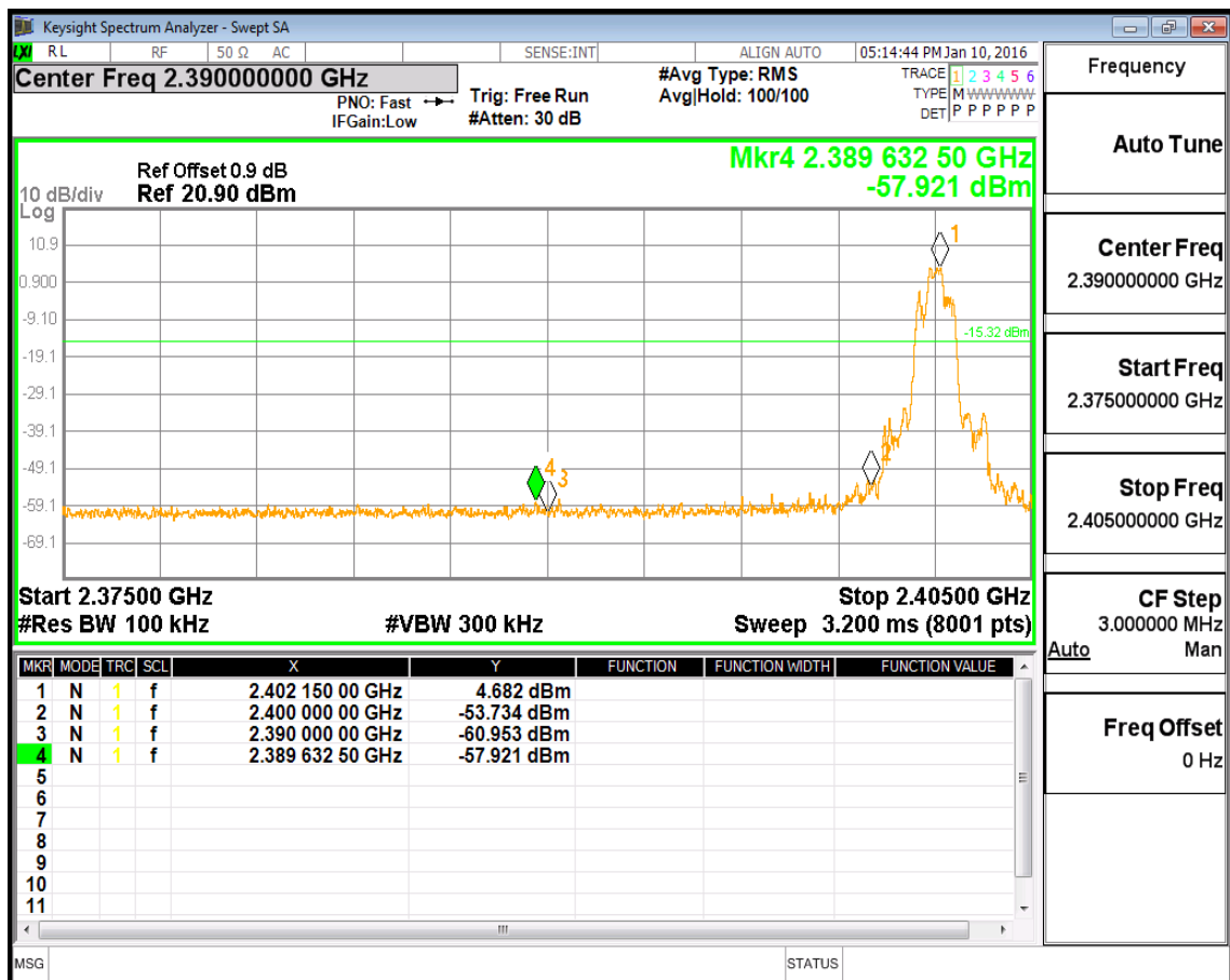
(Plot 4.9.2 D1: Left Band edge hopping off @ 8DPSK)
