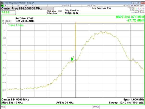
GSM_850_Lower_Band edge
