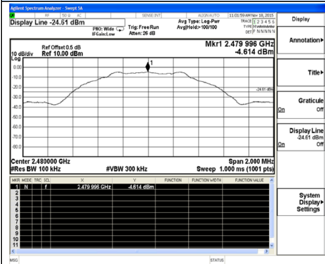
2479 - 2481 MHz
