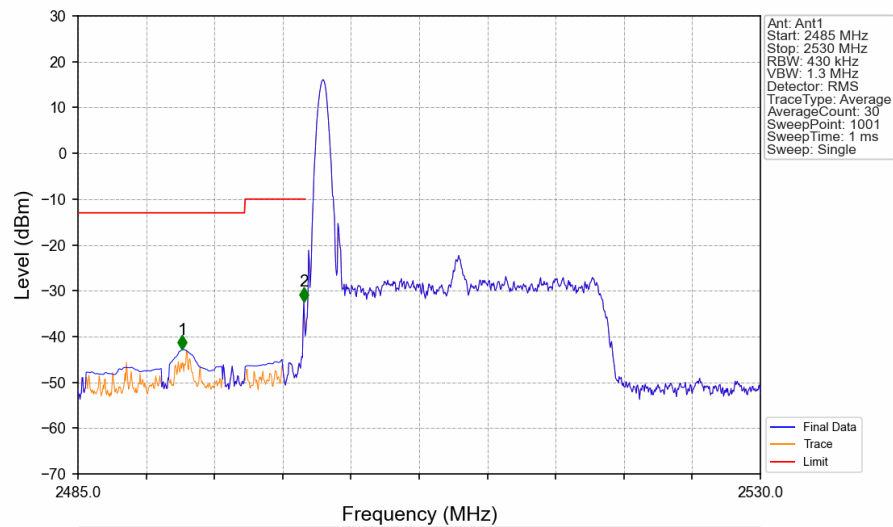
Band7_20MHz_QPSK_LCH_2510MHz_RB_1_0_NTNV
