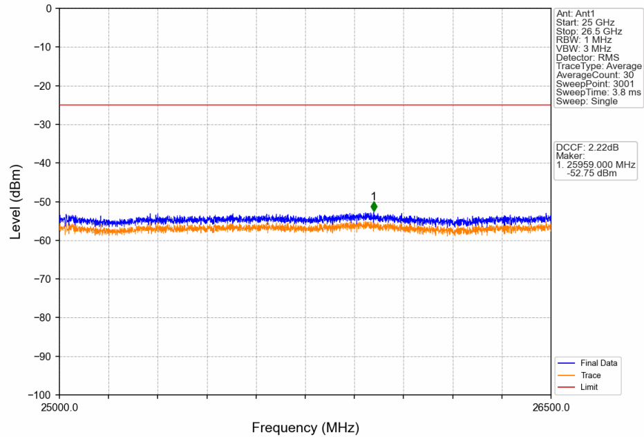
Band41_10MHz_QPSK_MCH_2605MHz_RB_1_0_NTNV
