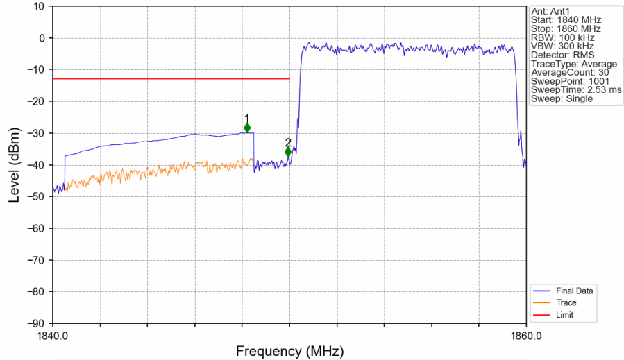
Band25_10MHz_QPSK_LCH_1855MHz_RB_50_0_NTNV
