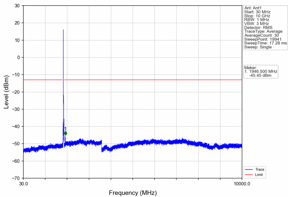
Band25_20MHz_QPSK_LCH_1860MHz_RB_1_0_NTNV
