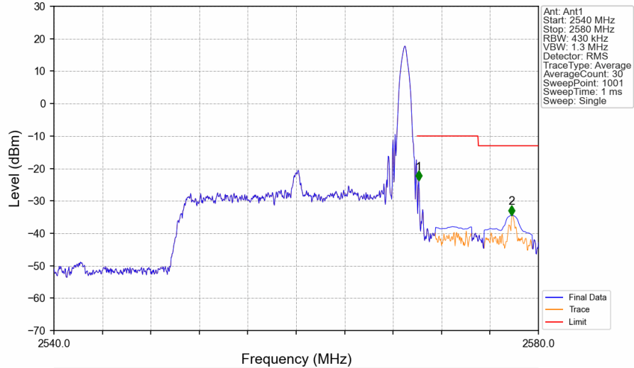
Band7_20MHz_QPSK_HCH_2560MHz_RB_1_99_NTNV
