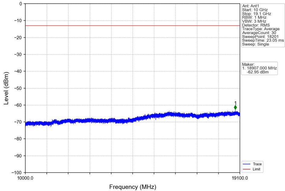
Band2_1.4MHz_QPSK_MCH_1880MHz_RB_1_0_NTNV
