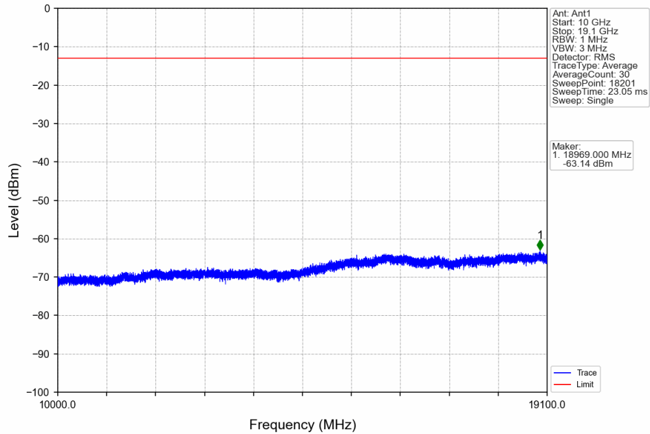
Band2_1.4MHz_QPSK_HCH_1909.3MHz_RB_1_0_NTNV
