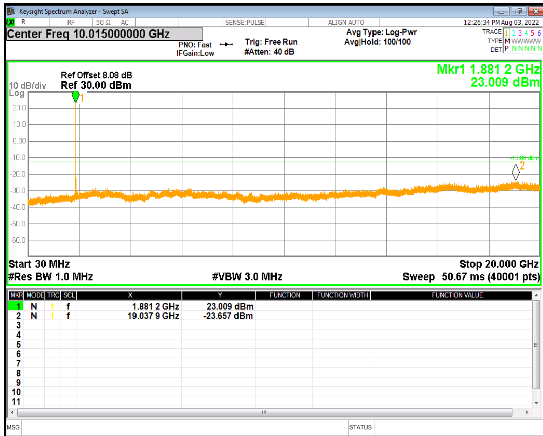
HSUPA Band2 Subtest4 Channel=9400
