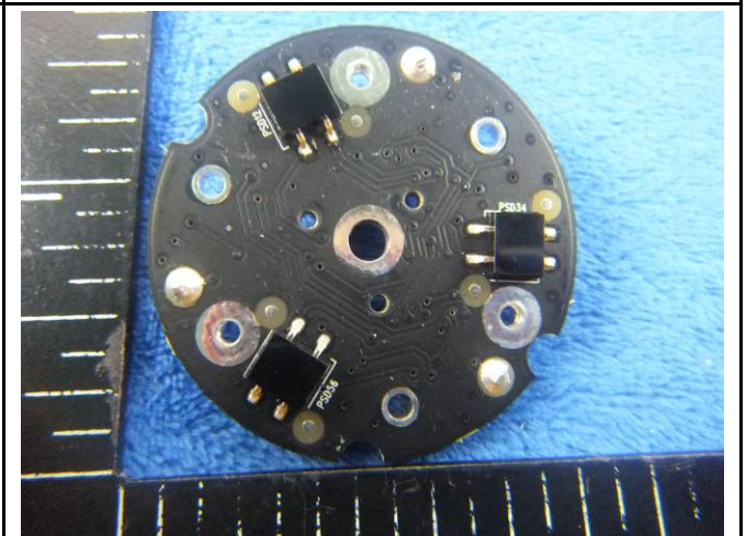
Mini Mainboard Board Bottom View
