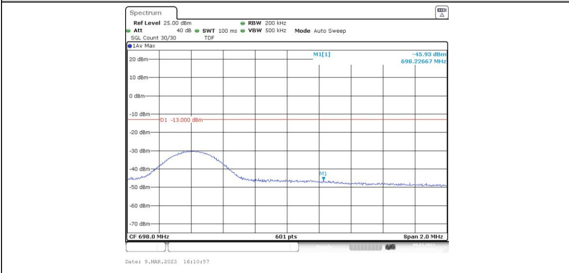
Band71-10MHz-QPSK-133422-1RB#49
