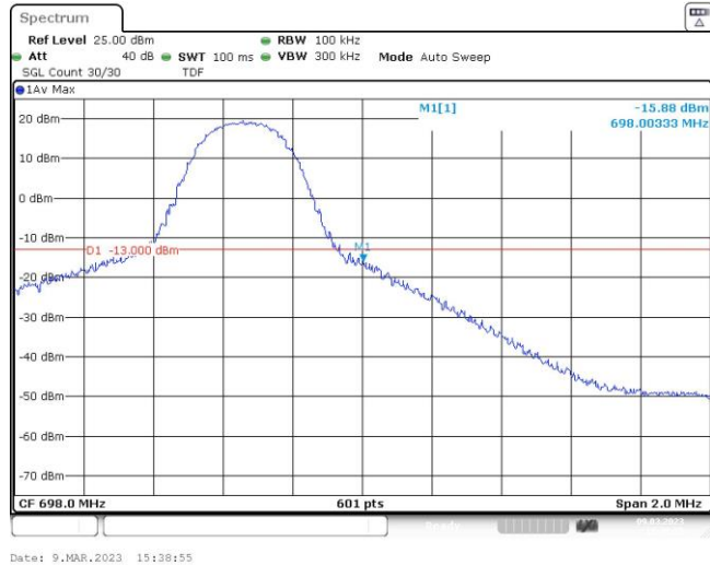
Band71-5MHz-QPSK-133447-25RB#0
