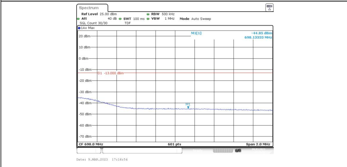
Band71-20MHz-16QAM-133372-1RB#99
