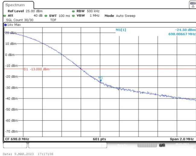
Band71-20MHz-QPSK-133372-100RB#0
