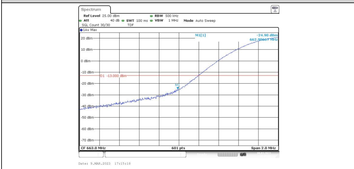
Band71-20MHz-QPSK-133222-1RB#99
