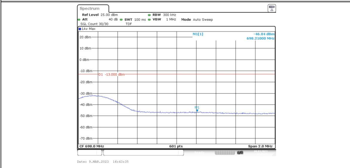
Band71-15MHz-QPSK-133397-1RB#74
