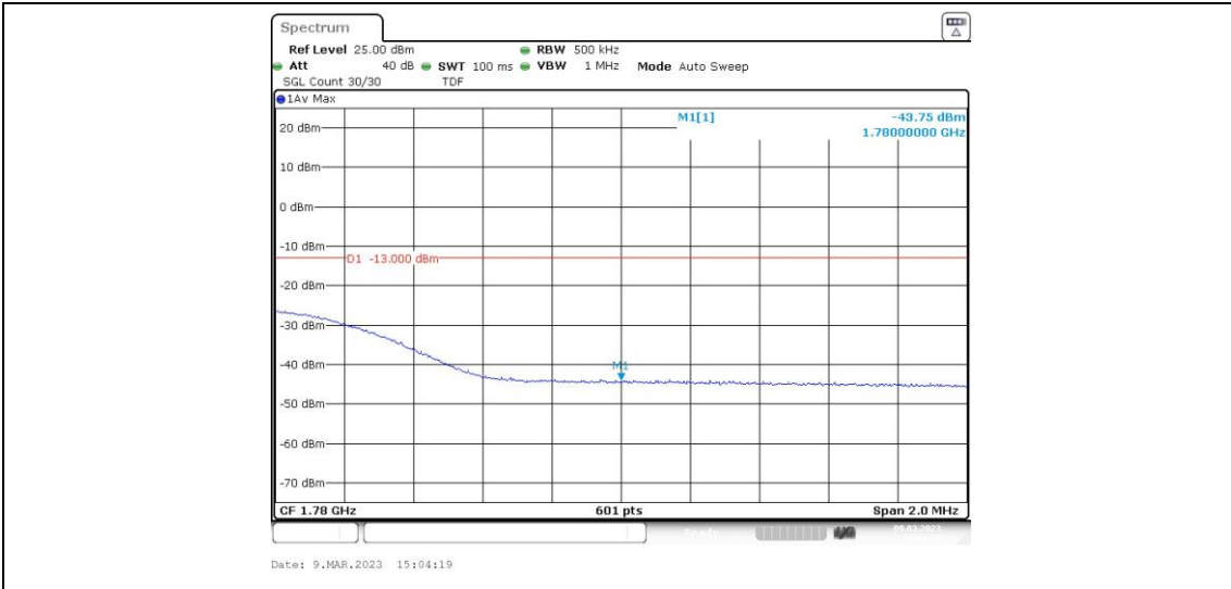
Band66-20MHz-QPSK-132572-1RB#99
