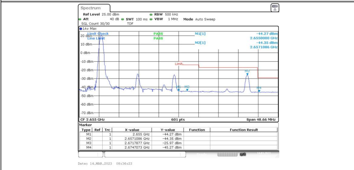
Band41-20MHz-QPSK-41140-1RB#99
