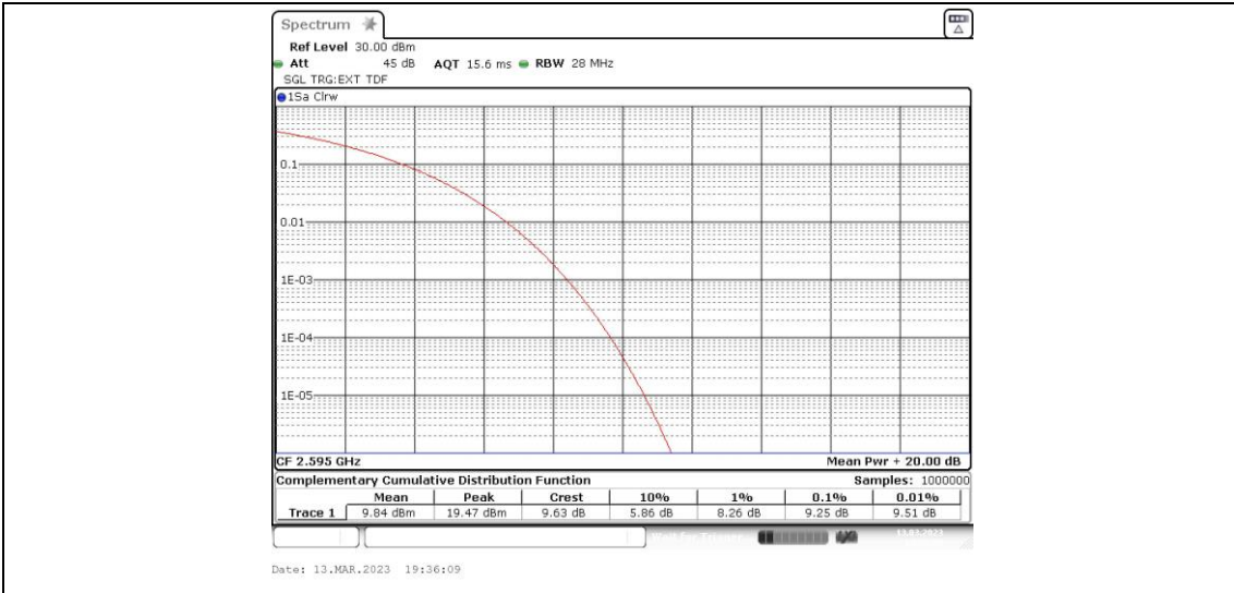
Band41-10MHz-QPSK-40640-50RB#0
