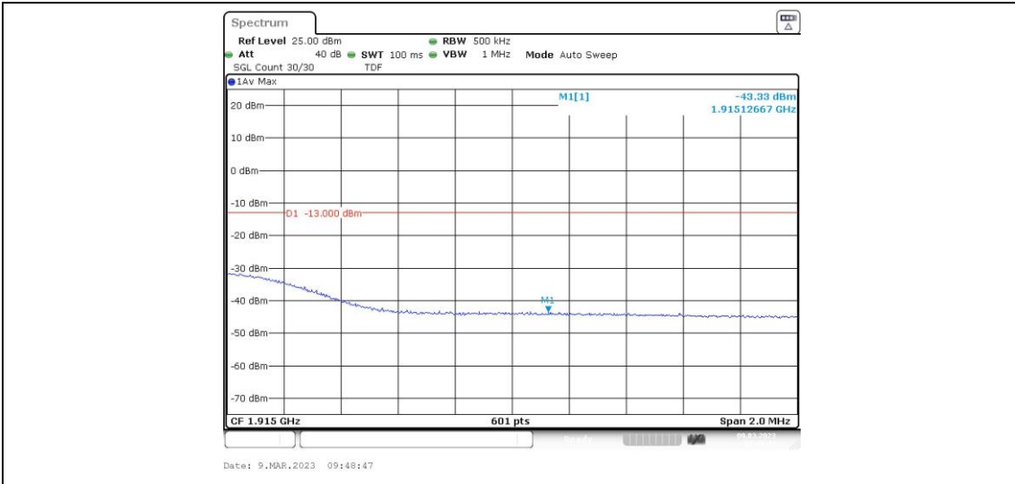
Band25-20MHz-16QAM-26590-1RB#99
