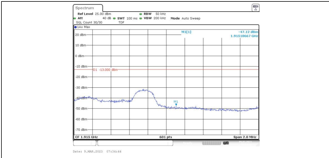
Band25-3MHz-QPSK-26675-1RB#14
