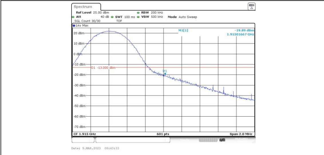
Band25-10MHz-QPSK-26640-50RB#0
