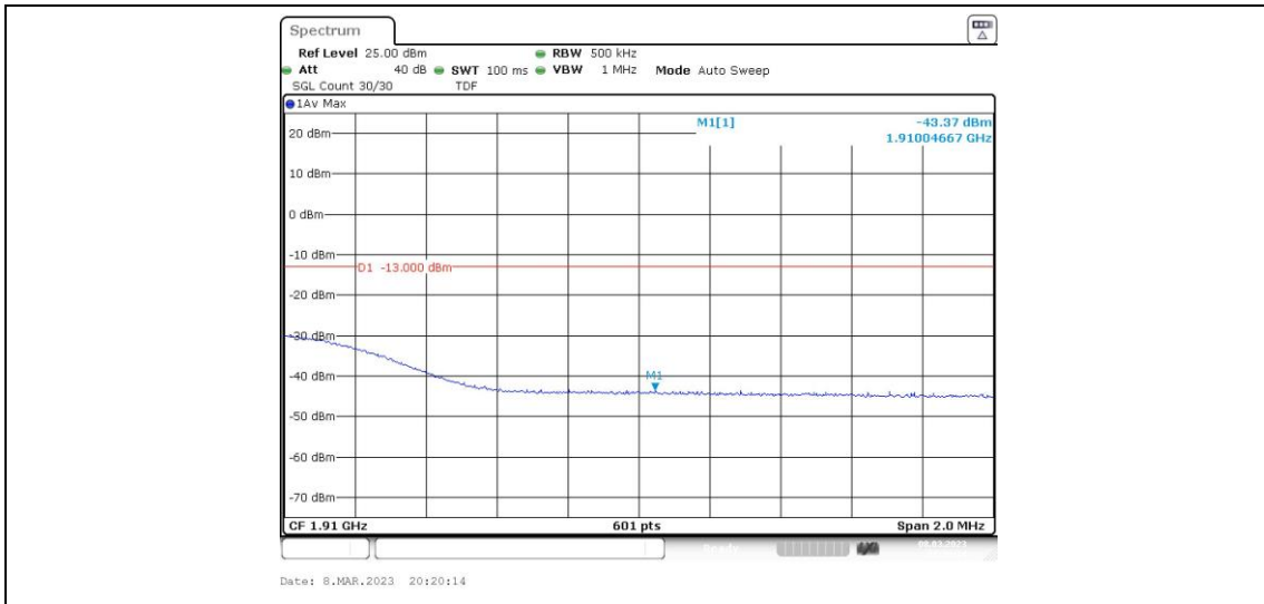
Band2-20MHz-QPSK-19100-1RB#99
