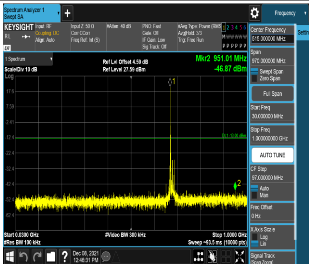
Band71-20MHz-QPSK-133372-1RB#0-Range1:30~1000MHz
