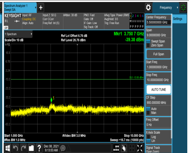
Band26-10MHz-QPSK-26740-1RB#0-Range2:1000~ 10000MHz
