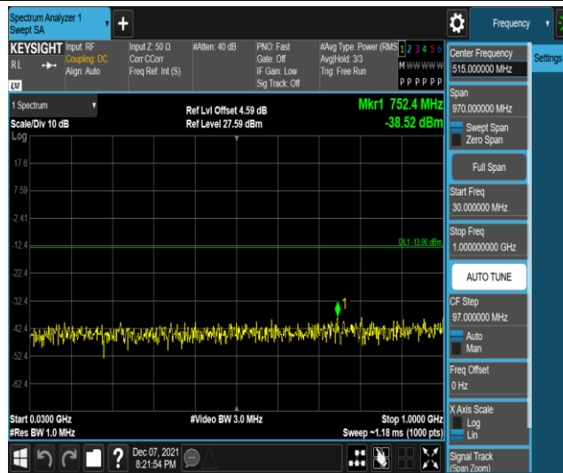
Band25-1.4MHz-16QAM-26365-1RB#0-Range1:30 ~1000MHz
