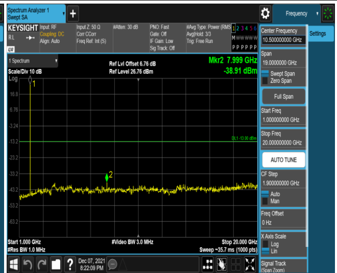
Band25-1.4MHz-16QAM-26365-1RB#0-Range2:1000 ~20000MHz
