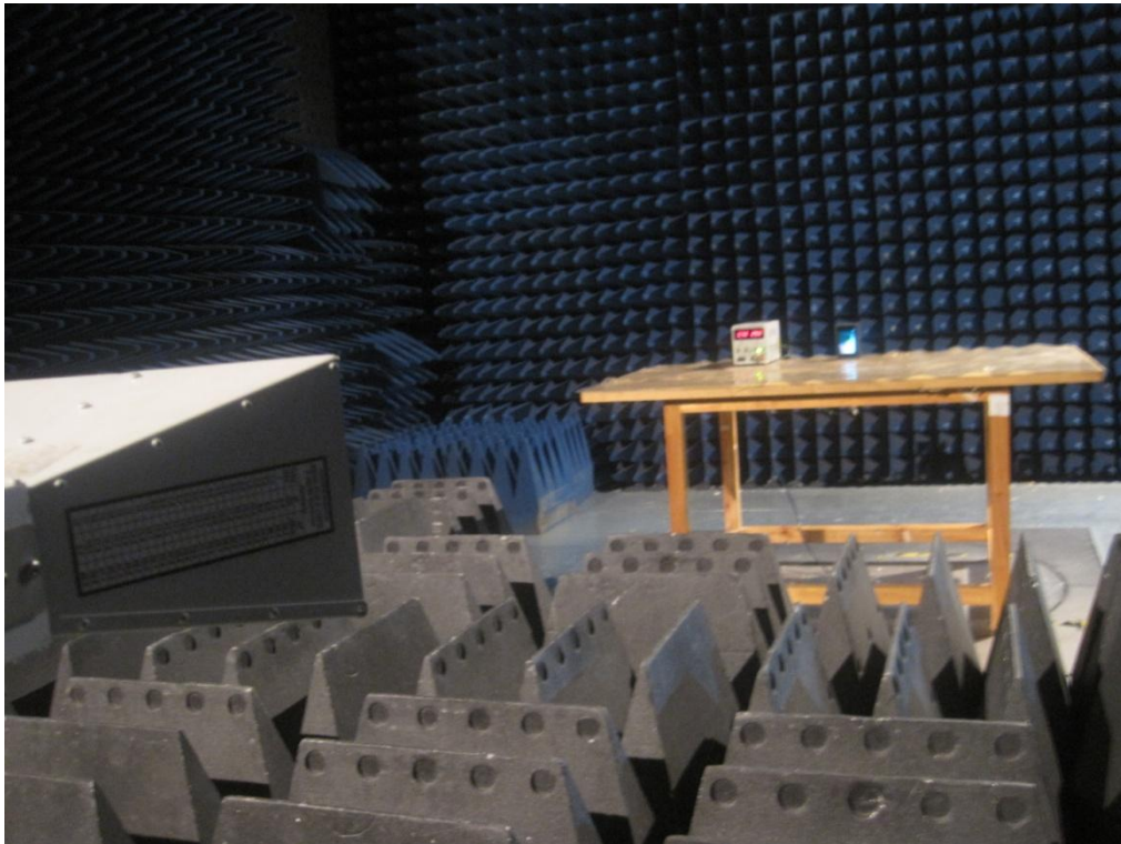
AV 5: Test frequency above 1GHz
