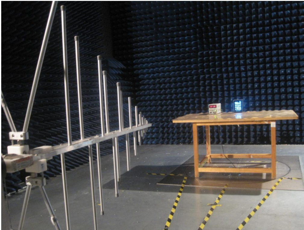
AV 7: Test frequency from 30MHz to 1GHz
