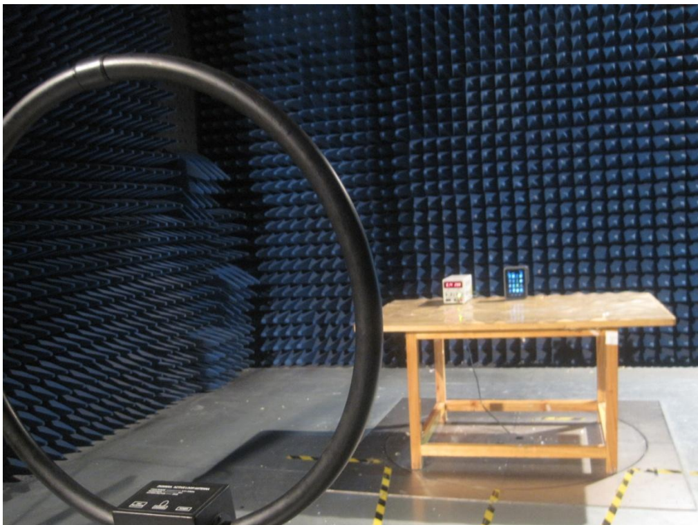
AV 7: Test frequency below 30MHz
