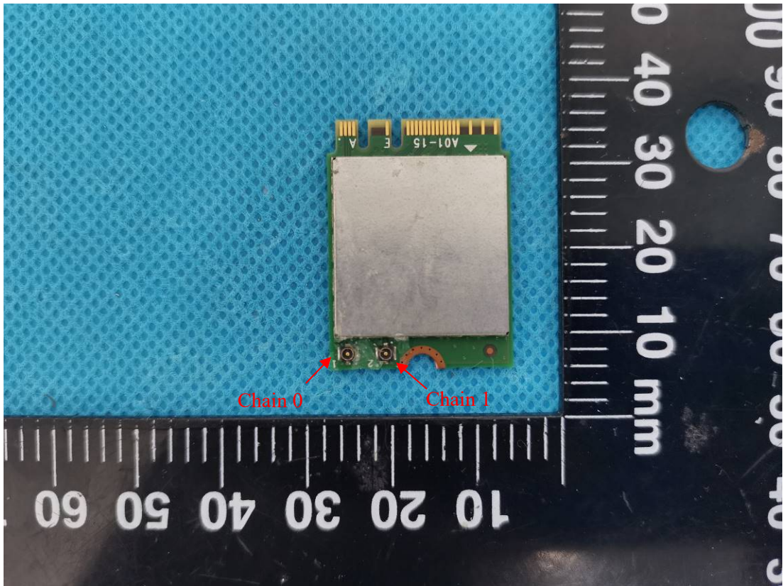
BT/WiFi Module
