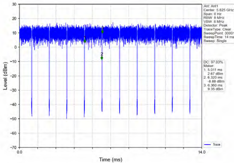
802.11n(HT20)_HCH_5825MHz_Ant1_NTNV
