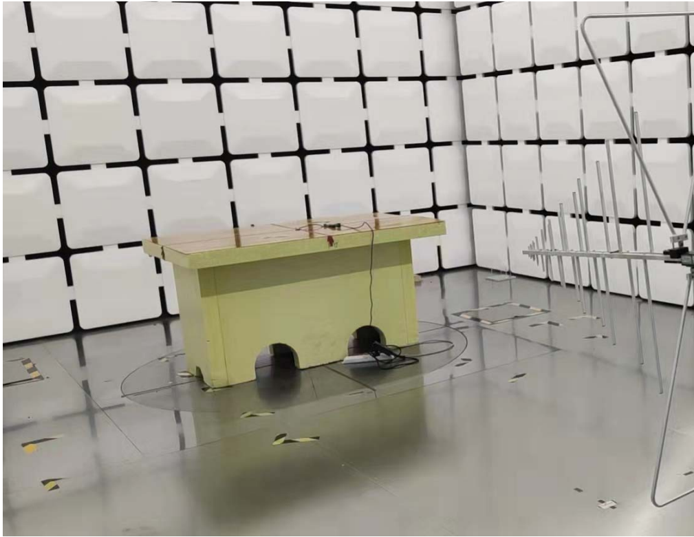
30MHz ~ 1GHz
