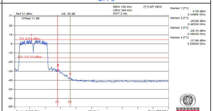
CH 9 Band edge
