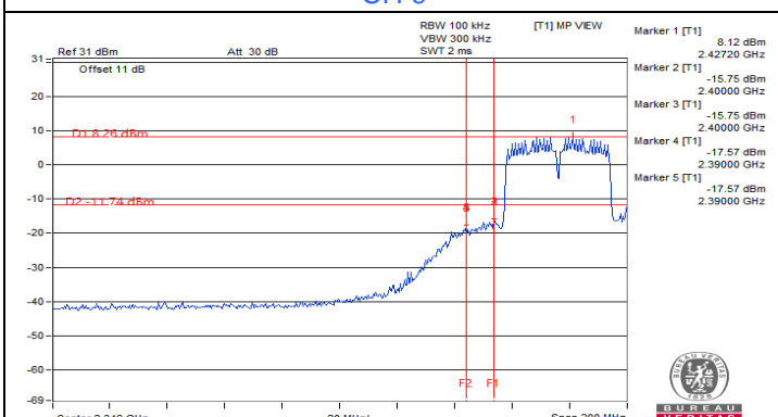
CH 3 Band edge
