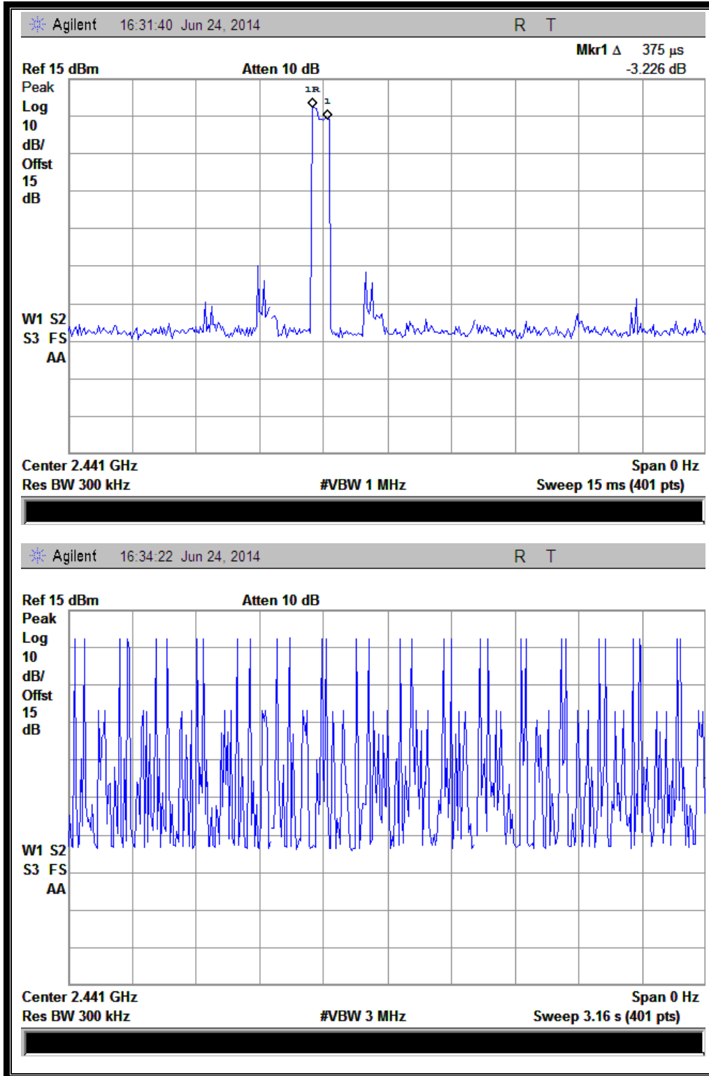
(Plot A: DH1 @ 1/4-DQPSK)
