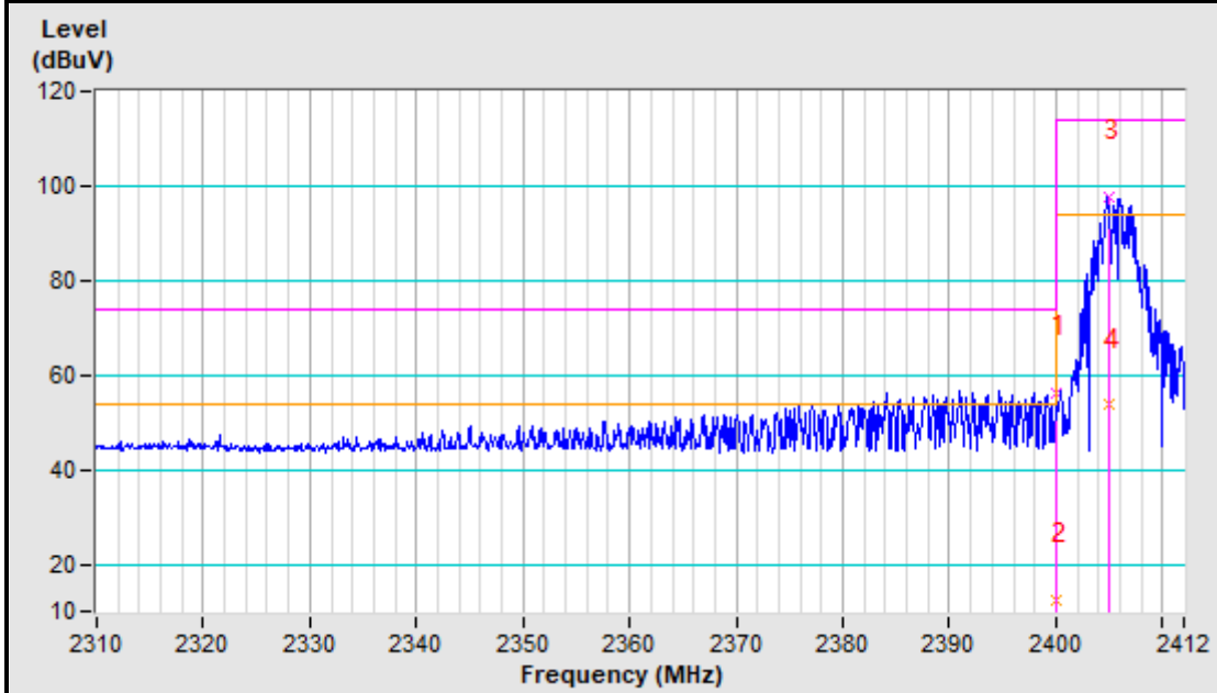
2405MHz Vertical
