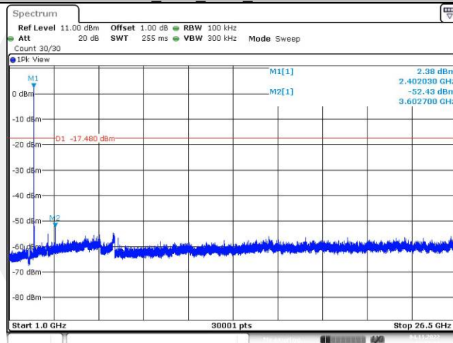
DH5_Ant1_2402_1000~26500
