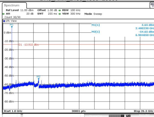
DH5_Ant1_2480_1000~26500
