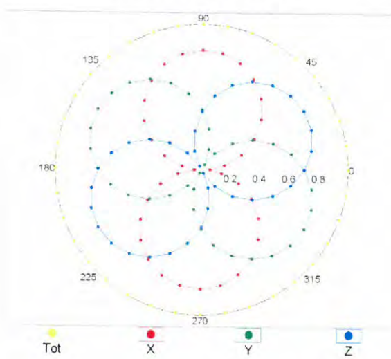
f=1800 MHz,R22
