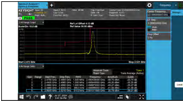
Band7 20MHz 16QAM 20850 1RB#0
