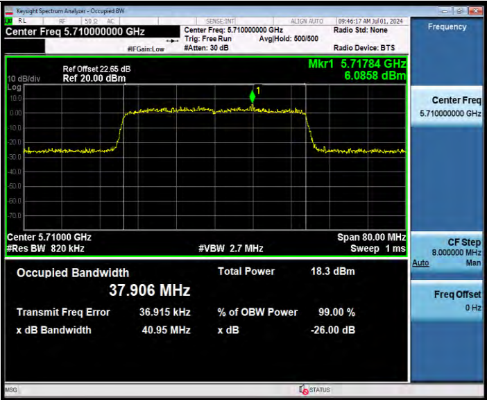
11AX40MIMO_Ant2_5710
