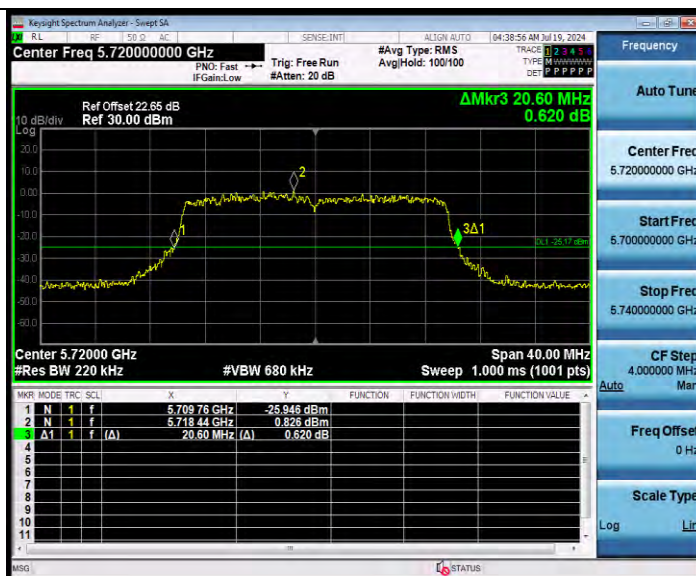
11AX20MIMO_Ant2_5720
