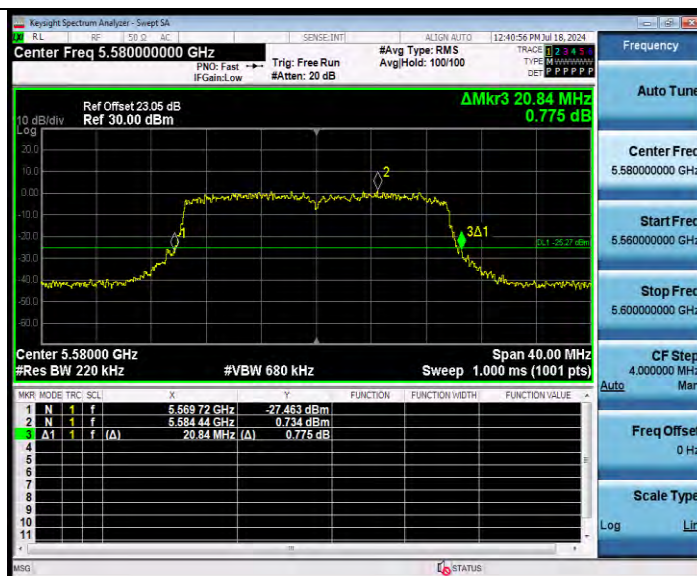
11AX20MIMO_Ant2_5580
