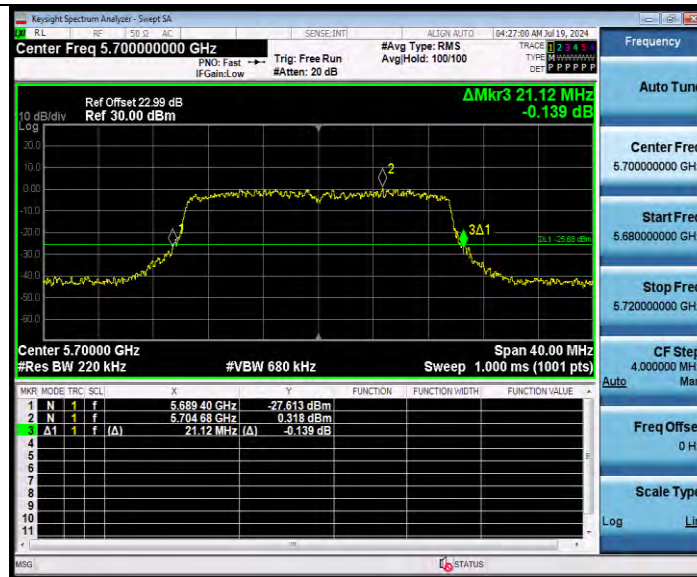
11AX20MIMO_Ant2_5700
