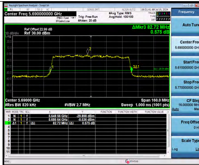
11AX80MIMO_Ant2_5690
