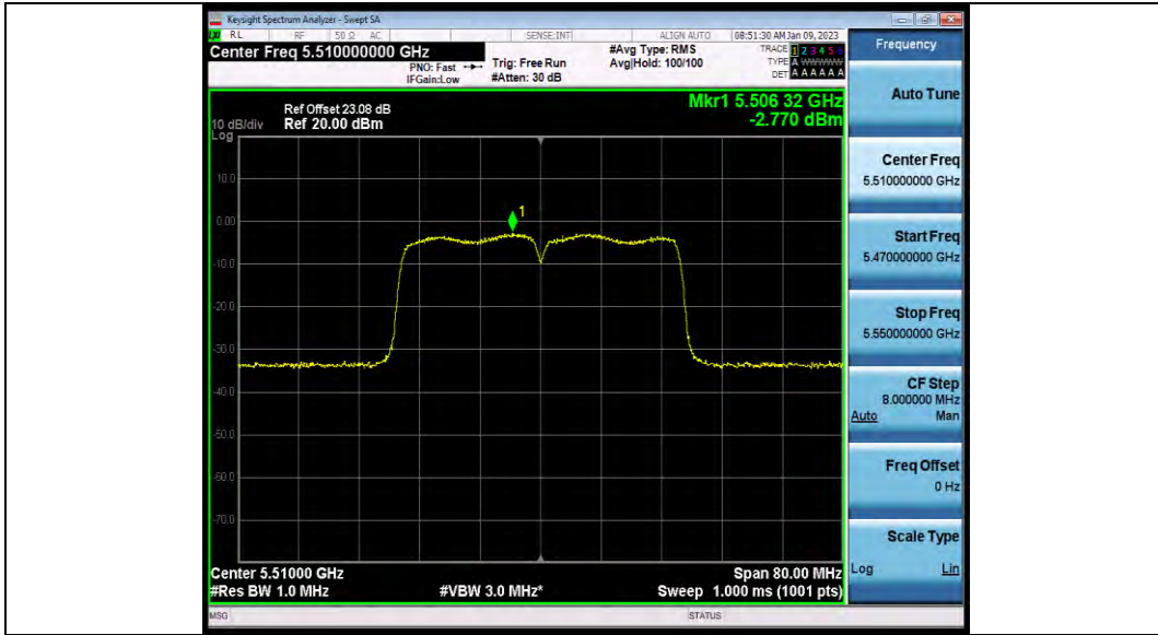
11N40MIMO_Ant2_5510
