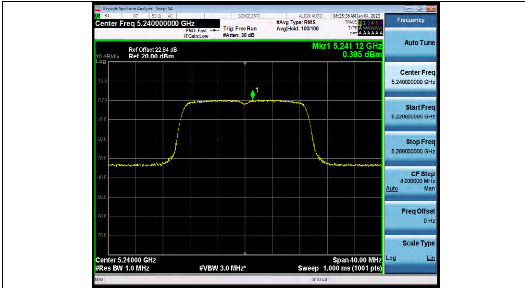
11N20MIMO_Ant2_5240
