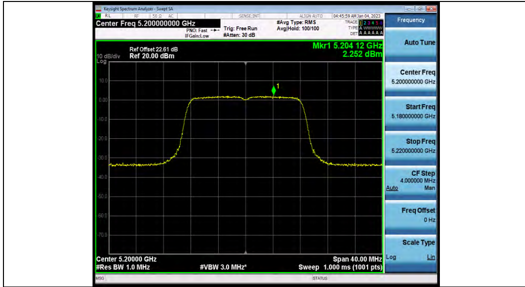
11A-CDD_Ant2_5200
