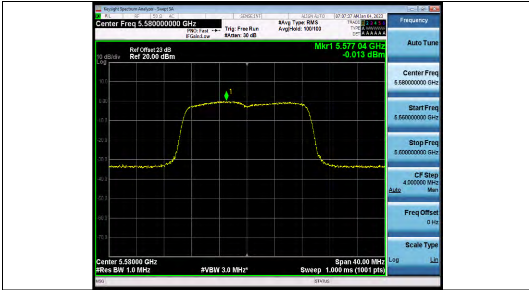
11N20MIMO_Ant2_5580
