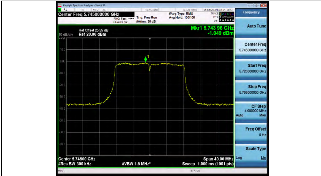
11A-CDD_Ant2_5745
