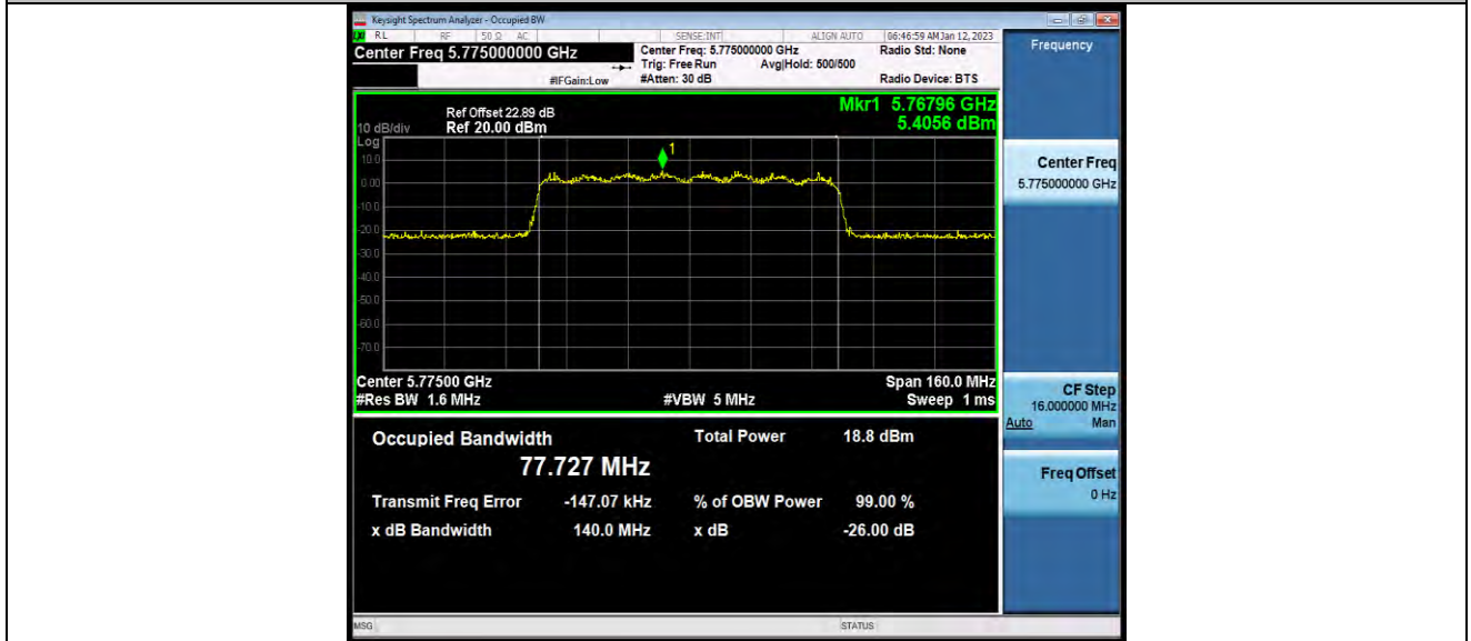
11AX80MIMO_Ant2_5775
