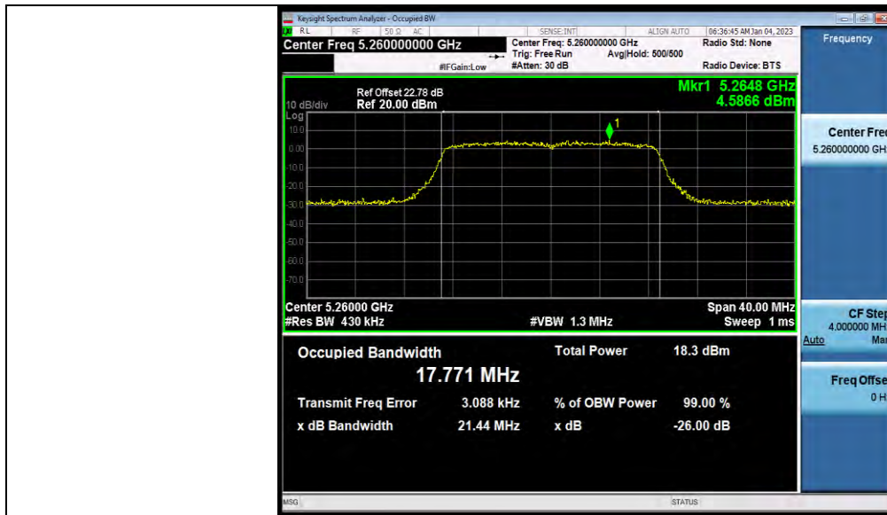
11N20MIMO_Ant2_5260
