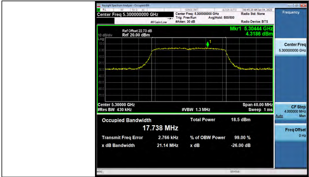
11N20MIMO_Ant2_5300
