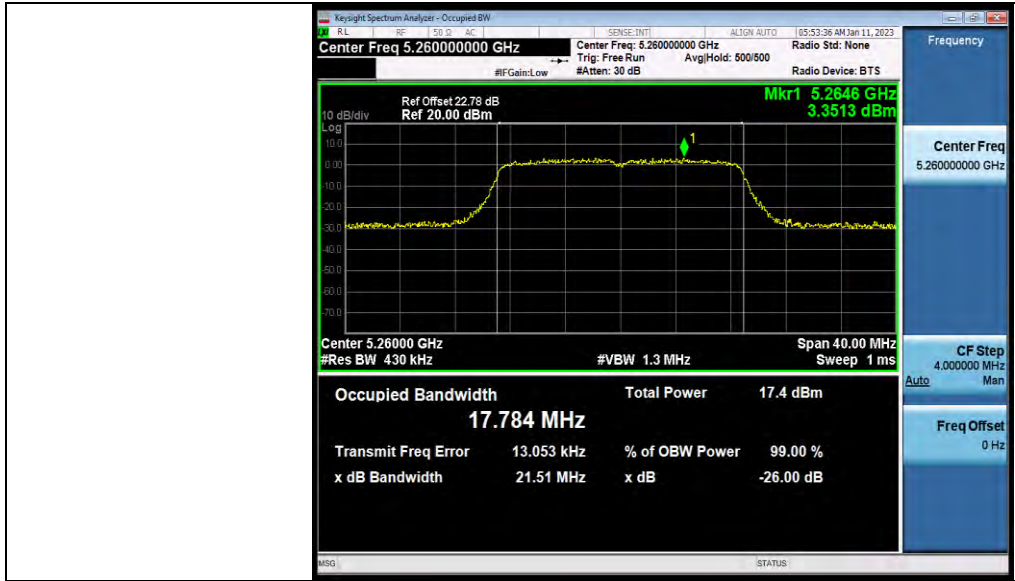
11AC20MIMO_Ant2_5260
