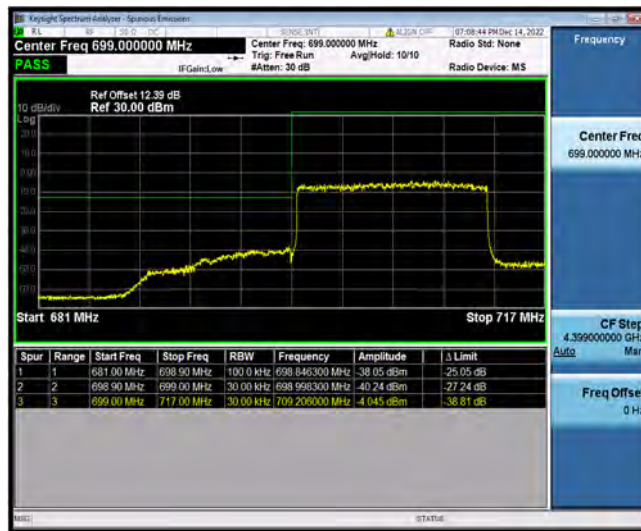
N12-15MHz-QPSK-141700-1RB#74
