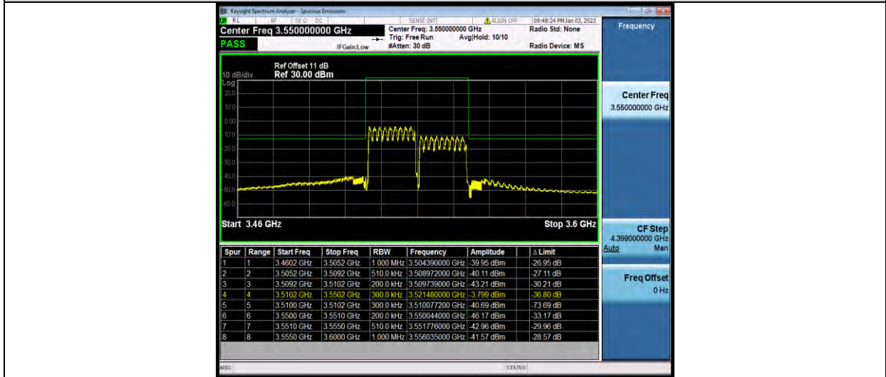
42-42-20MHz-20MHz-QPSK-QPSK-42792-42990-1RB#0-1RB#99
