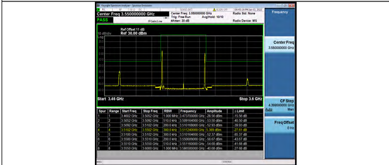
42-42-20MHz-20MHz-16QAM-16QAM-42792-42990-1RB#99-1RB#0
