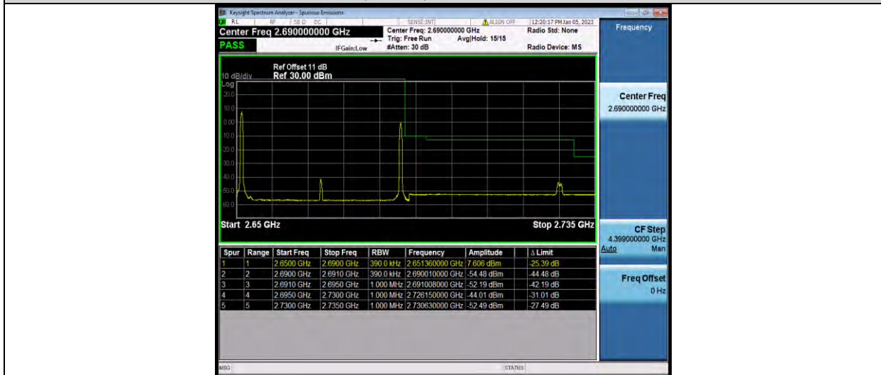
41-41-20MHz-20MHz-QPSK-QPSK-41292-41490-1RB#99-1RB#0
