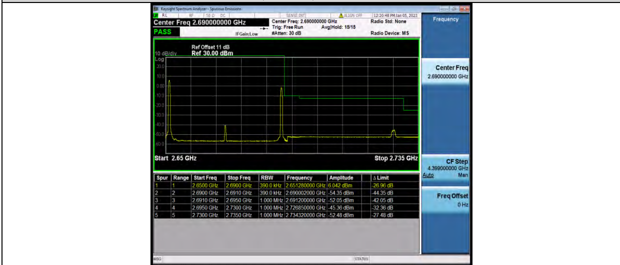
41-41-20MHz-20MHz-16QAM-16QAM-41292-41490-1RB#99-1RB#0
