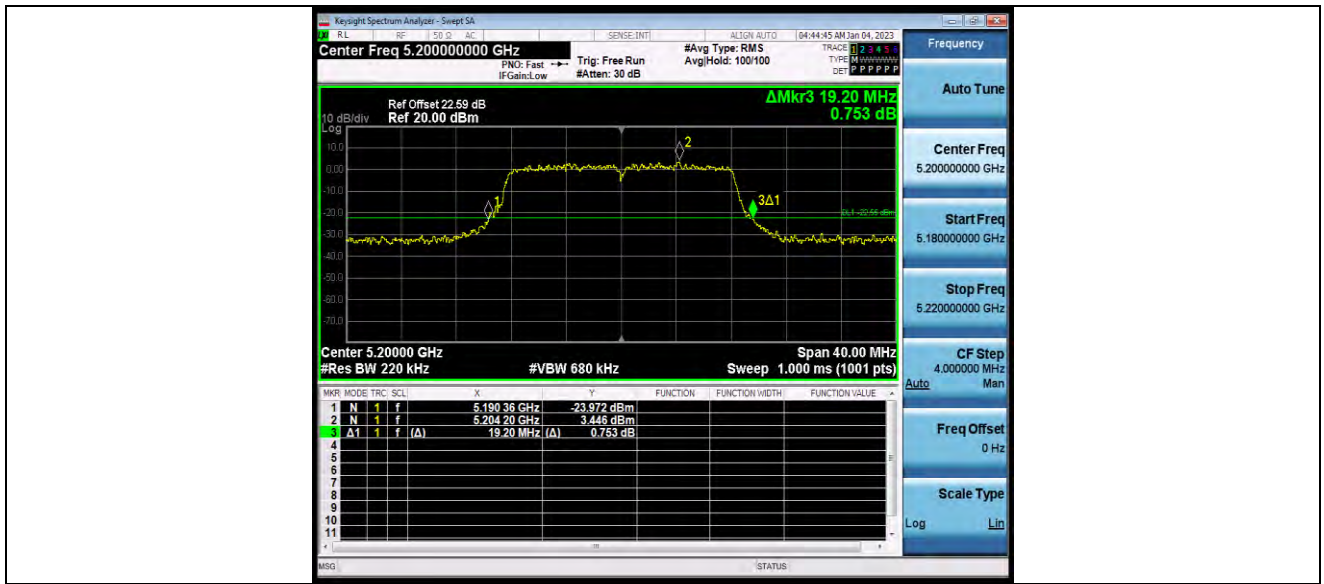
11A-CDD_Ant2_5200
