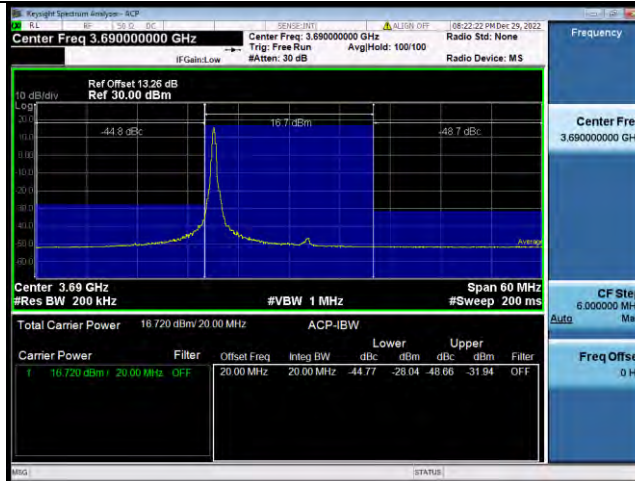
Band48-20MHz-QPSK-56640-1RB#99
