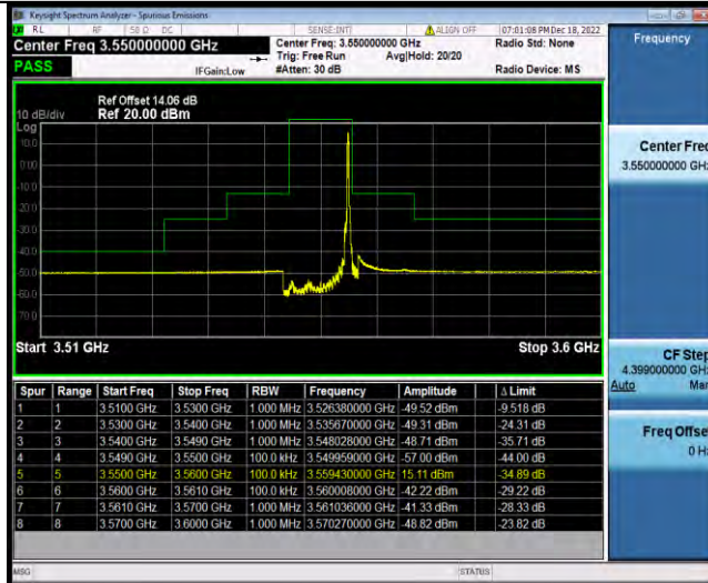
Band48-10MHz-QPSK-55290-50RB#0
