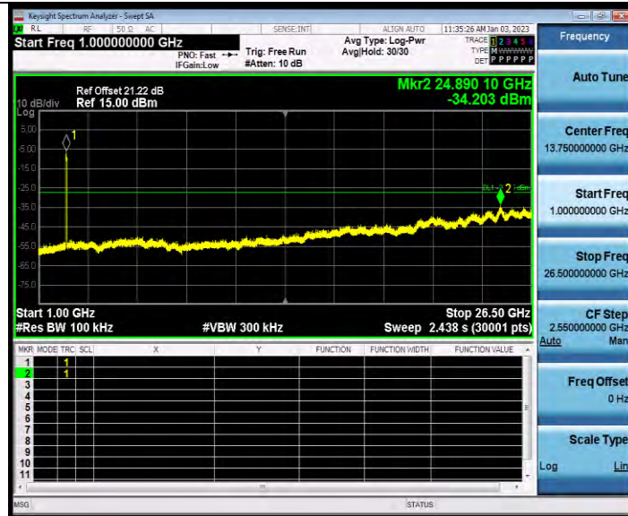
11AX40MIMO_Ant2_2437_0~Reference
