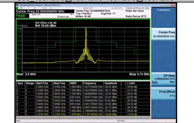
20MHz-20MHz_QPSK@QPSK-QPSK@QPSK_55891-56 089 1RB#99@100RB#0-1RB#0@100RB#0
